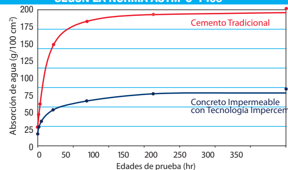
GRÁFICA DE ABSORCIÓN POR CAPILARIDAD SEGÚN LA NORMA ASTM-C-1403
